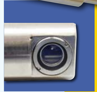
TV-Endoskop mit Wasser- und Schweißfiltereinbauten Objektiv-Blickrichtung 90° mit wechselbarem Saphir-Schutzglas und Freiblasvorrichtung
